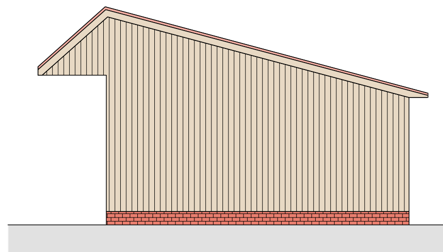
Ansicht Süd
