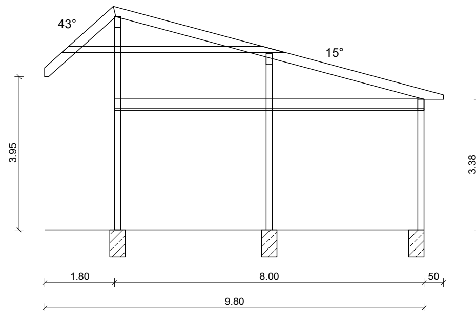
Schnitt A-A
