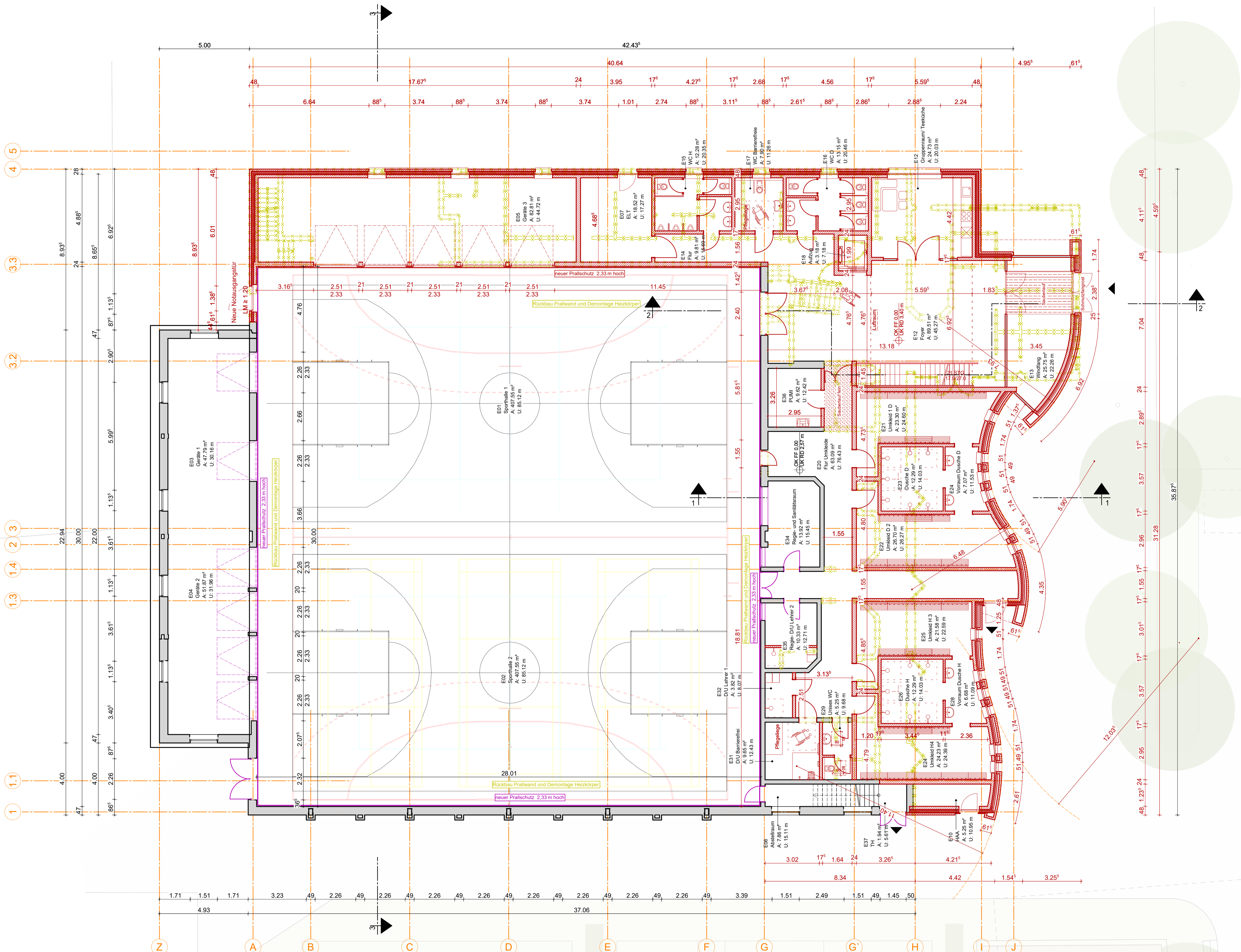
ERDGESCHOSS M 1:100
