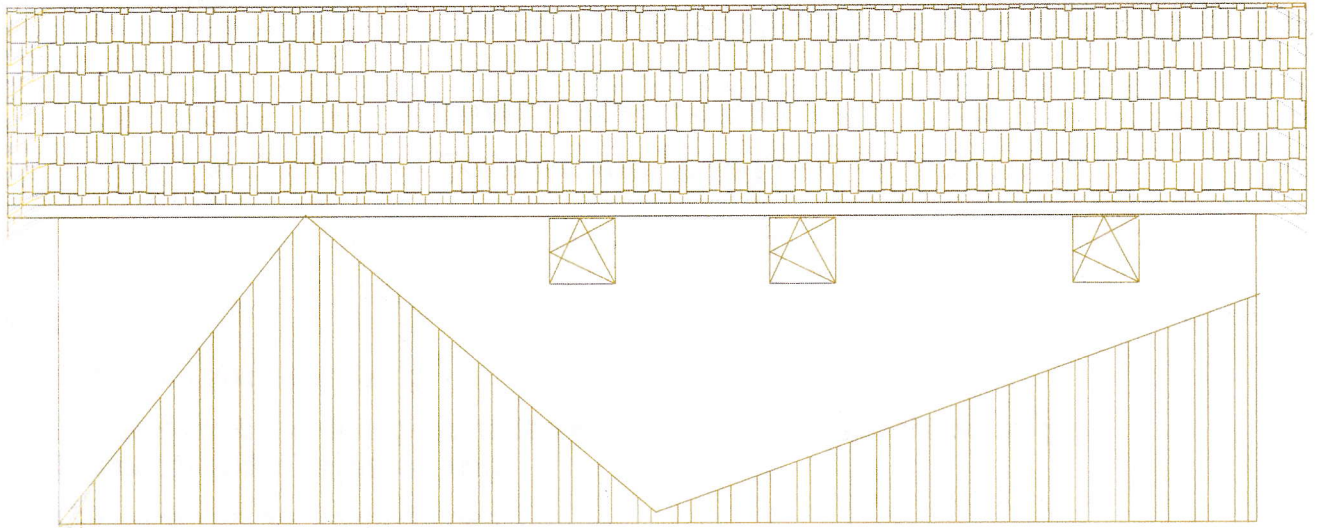
Ansicht Süd
