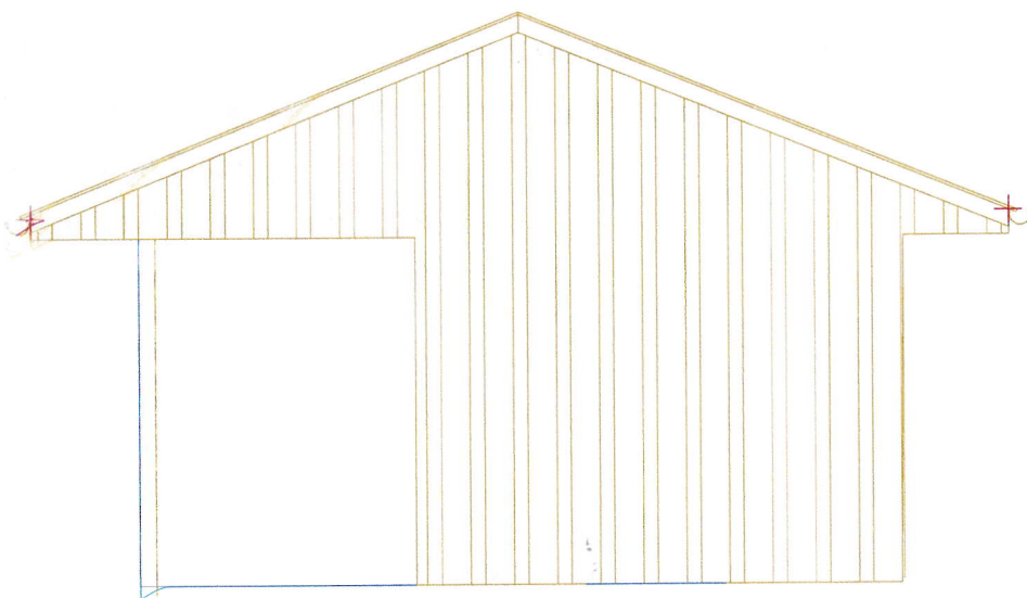
Ansicht Westen
